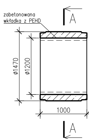
PRZEKRÓJ B-B
